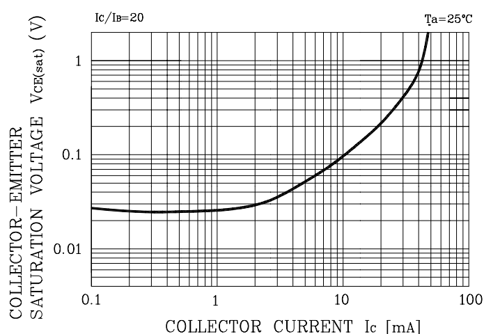
Fig. 2 V_{CE(SAT)} - I_C
