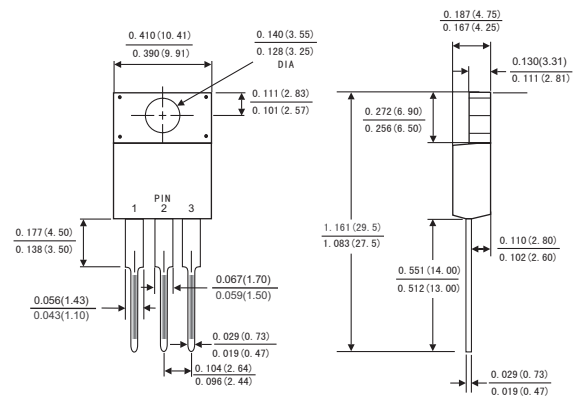
ITO-220AB
