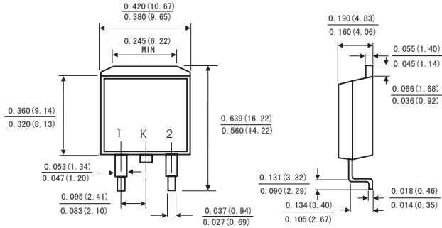
TO-263
