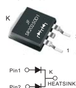
TO-263
