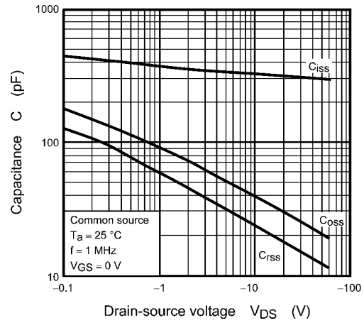
Fig. 8.8 C - V_{DS}
