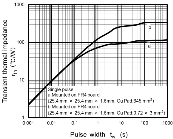
Fig. 8.11 r_{th} - t_w
