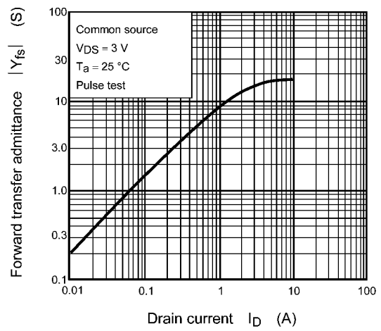
Fig. 8.8 |Y_{fs}| - I_D
