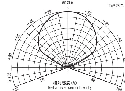
■指向特性
