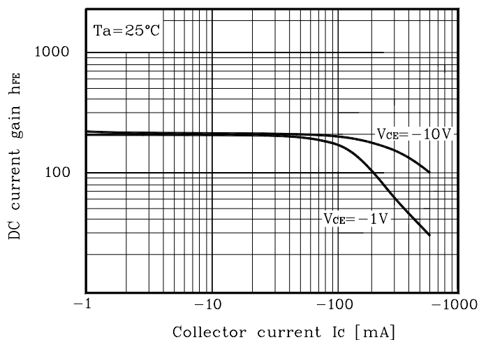
Fig. 5 h_{FE} - I_C
