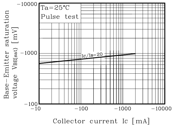
Fig. 6 V_{BE(sat)} - I_C
