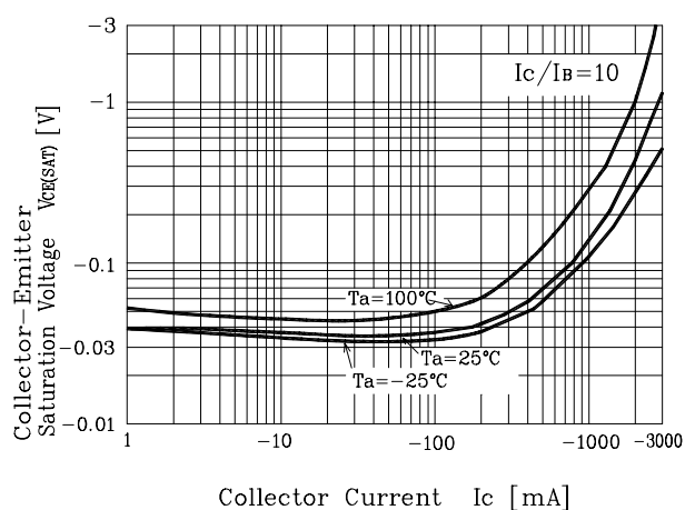
Fig. 4 V_{CE(sat)} - I_C
