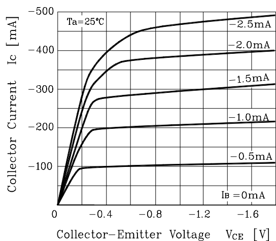
Fig. 3 I_C - V_{CE}
