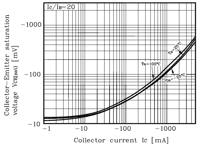
Fig. 4 V_{CE(sat)} - I_C
