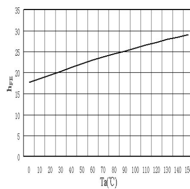
h_{FE} - T_a
