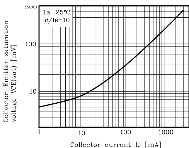
Fig. 1 V_{CE(sat)} - I_C
