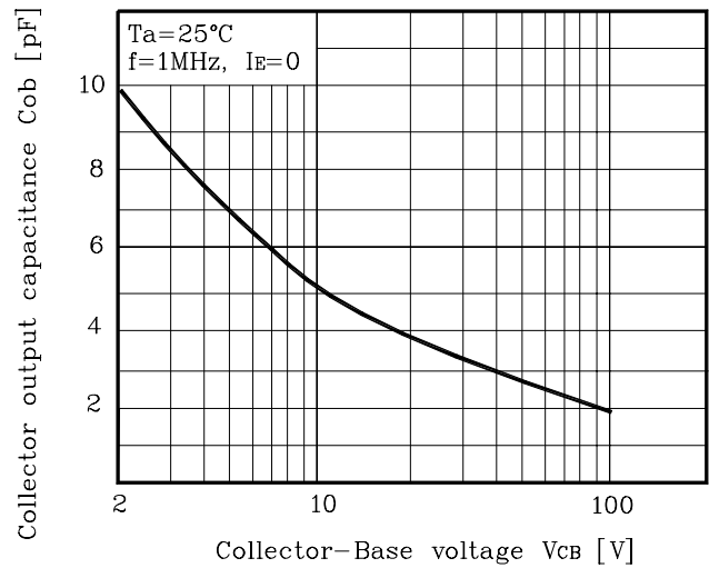
Fig. 1 C_{ob}-V_{CB}
