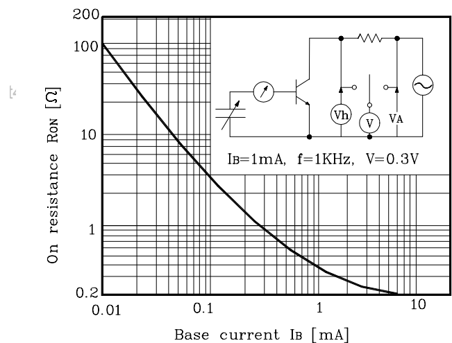
Fig. 4 R_{ON}-I_B
