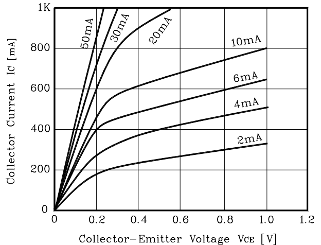
Fig. 6 I_C - V_{CE}
