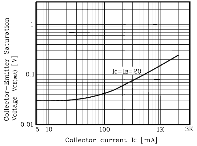
Fig. 2 V_{CE} - I_C
