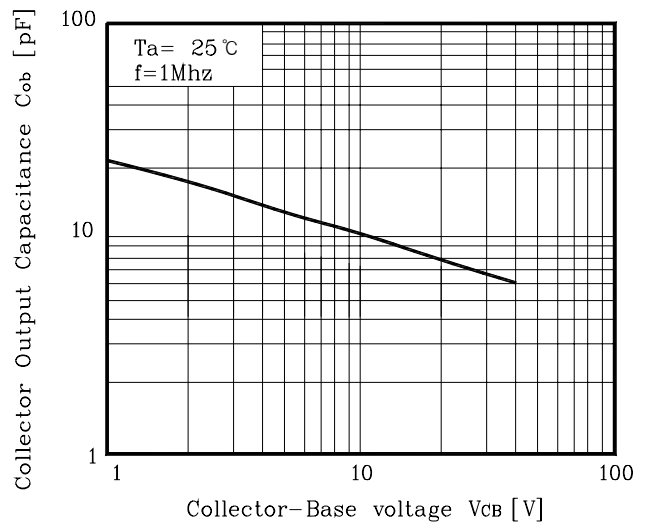
Fig. 10 C_{ob} - V_{CB}
