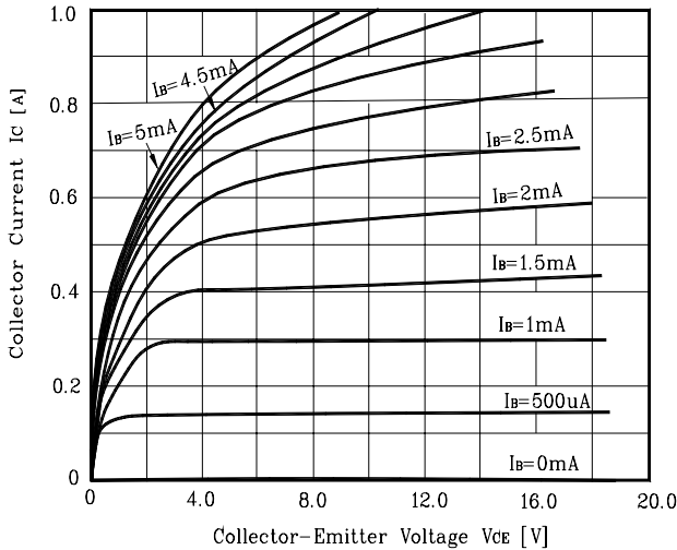
Fig. 5 I_C - V_{CE}
