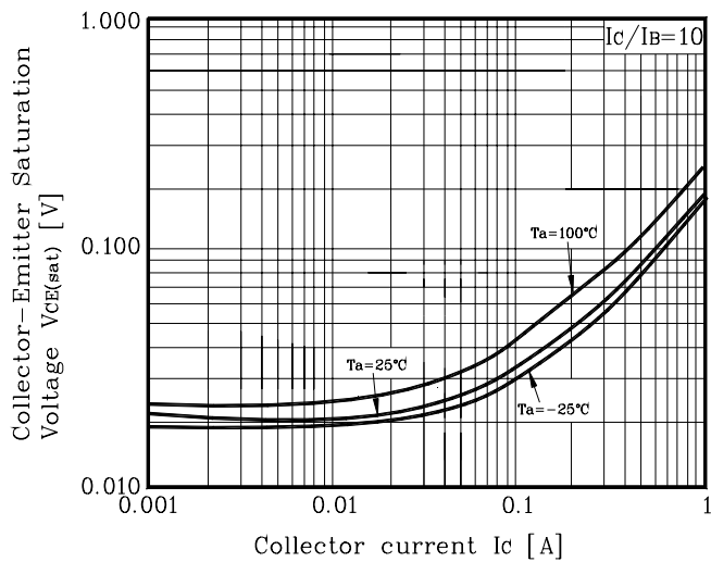
Fig. 3 V_{CE(sat)} - I_C
