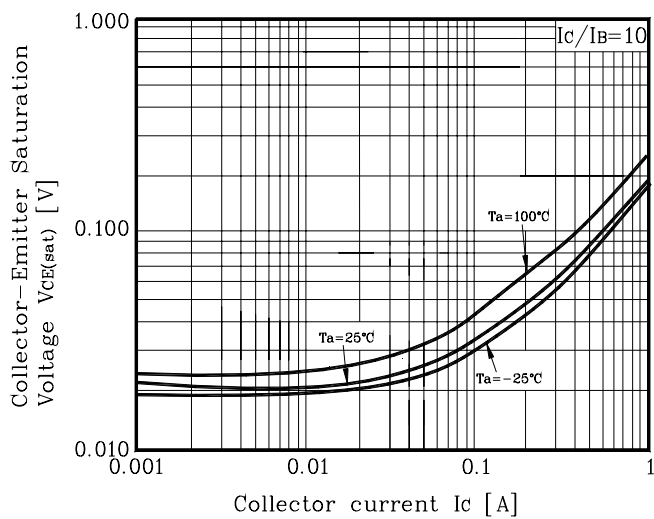
Fig. 3 V_{CE(sat)} - I_C
