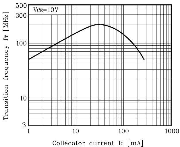
Fig. 5 f_T - I_C
