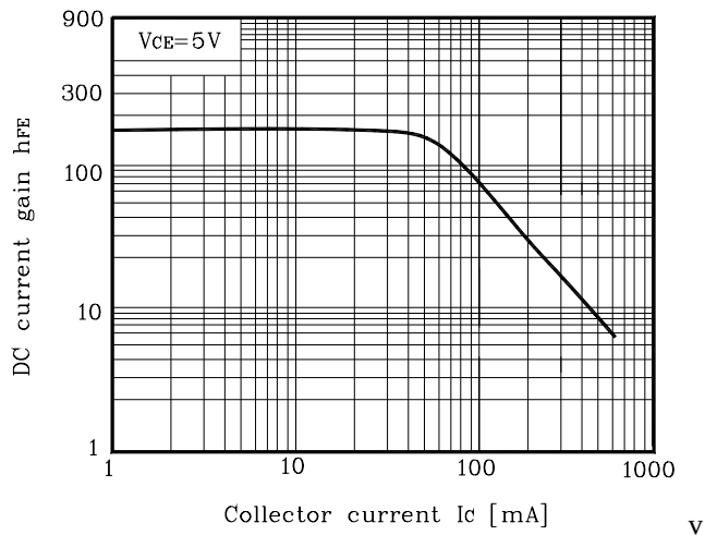
Fig. 3 h_{FE} - I_C
