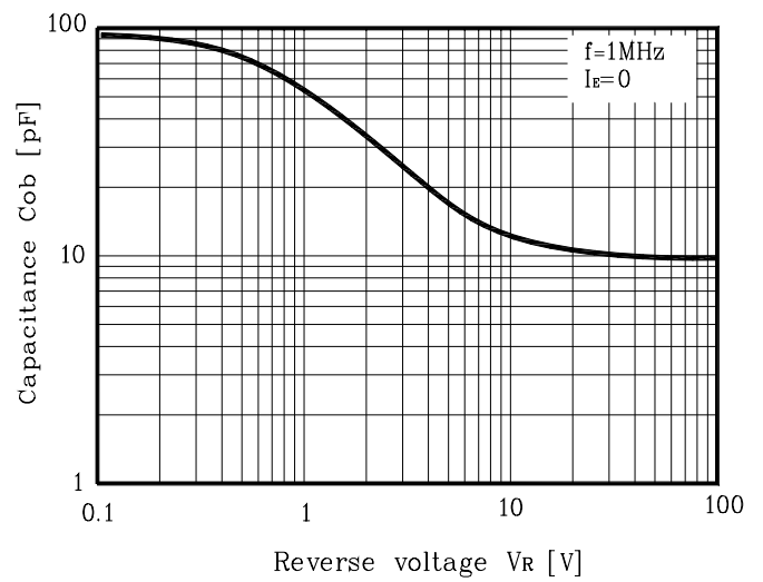
Fig. 4 C_{ob} - V_R
