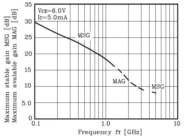
Fig. 7 MSG,MAG-f T
