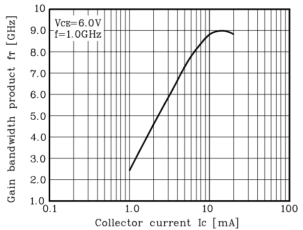
Fig. 4 f_T-I_C
