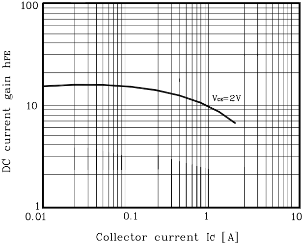
Fig. 3 h_{FE} - I_C
