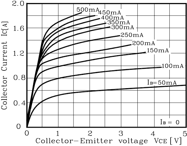
Fig. 1 I_C - V_{CE}
