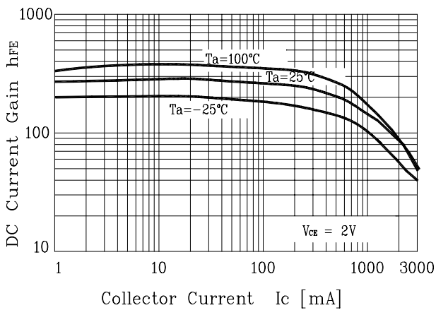
Fig. 5 h_{FE} - I_C
