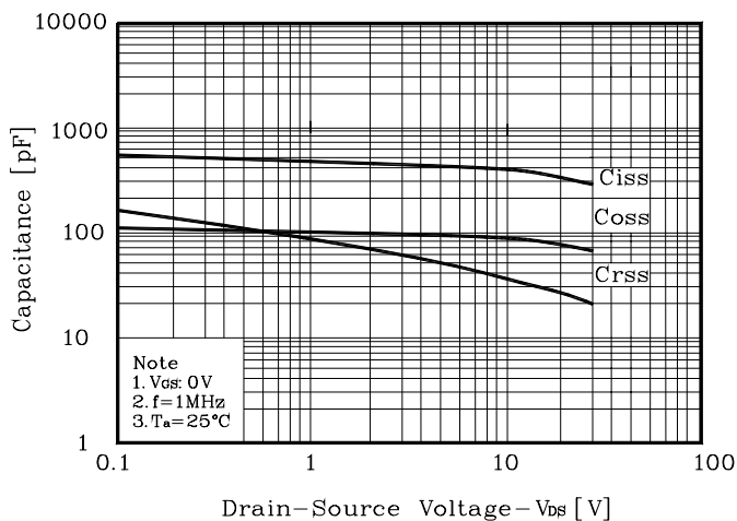
Fig. 5 Capacitance - V_{DS}
