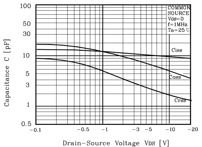
Fig6 C - V_{DS}
