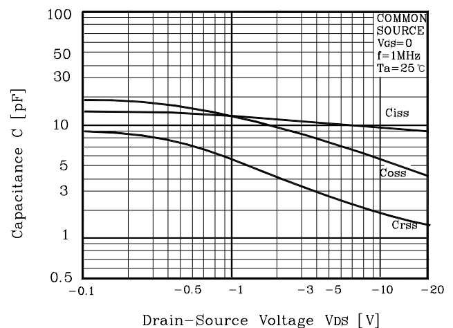
Fig6 C - V_{DS}
