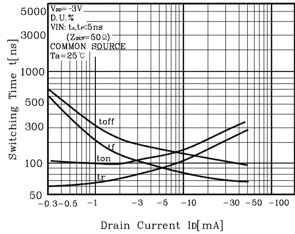
Fig8 t - I_D
