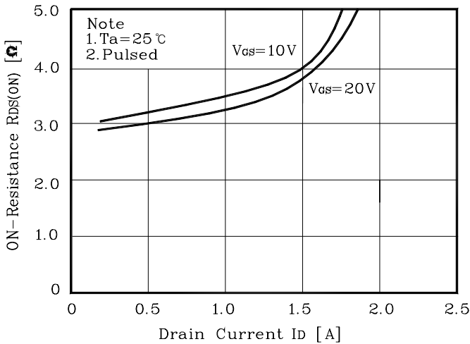
Fig. 3 R_{DS(on)} - I_D
