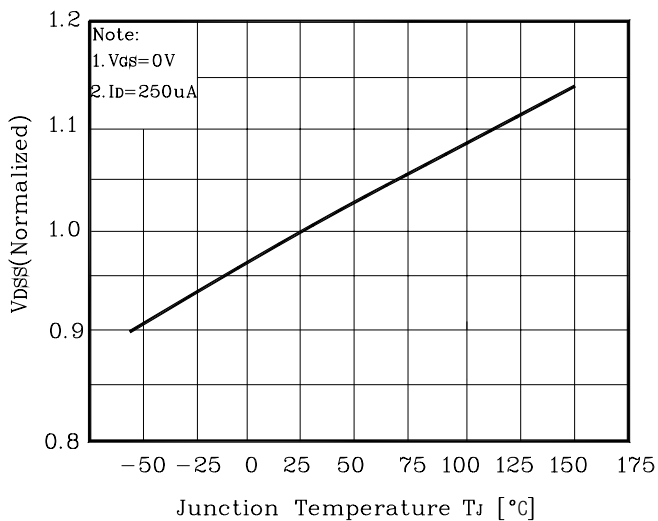
Fig. 7 V_{DSS} - T_J
