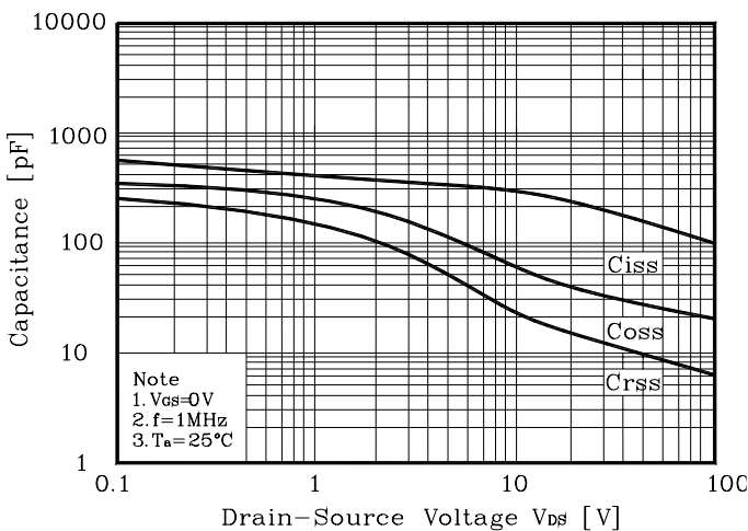
Fig. 5 Capacitance - V_{DS}
