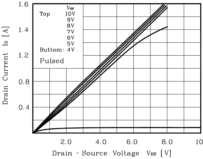
Fig. 1 I_D - V_{DS}
