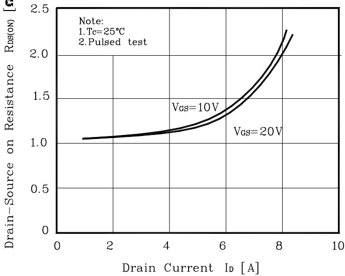
Fig. 3 R_{DS(on)} - I_D
