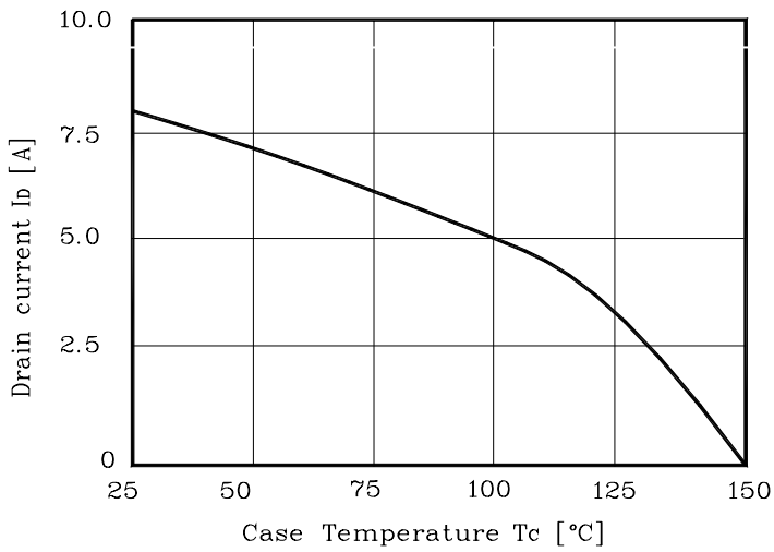
Fig. 9 I_D - T_C
