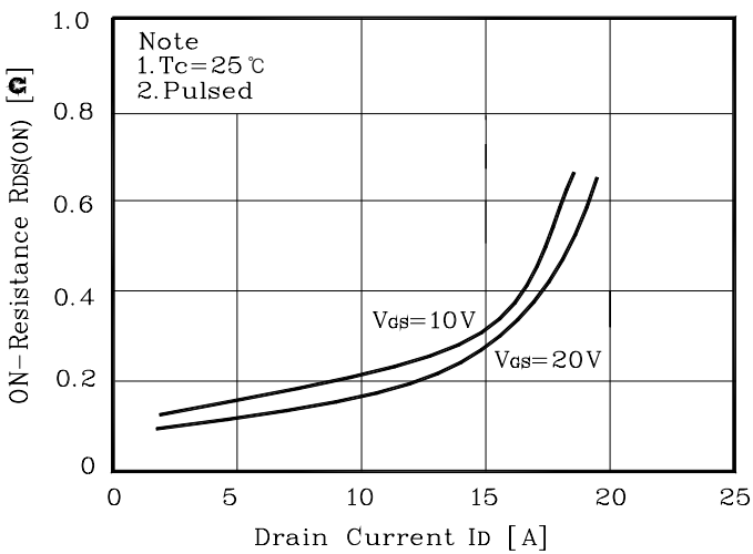
Fig. 3 R_{DS(on)} - I_D
