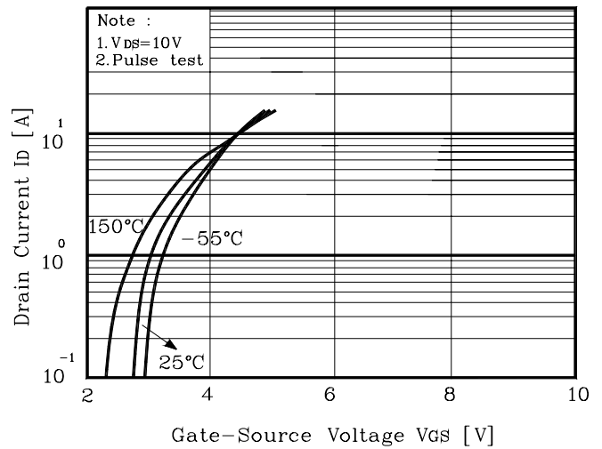
Fig. 2 I_D - V_{GS}
