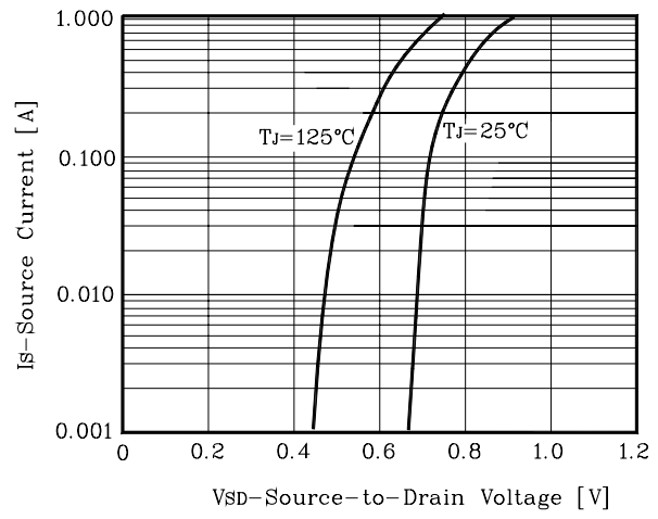
Fig. 8 I_S - V_{SD}
