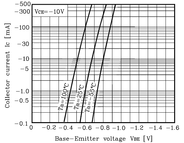
Fig. 2 I_C - V_{BE}
