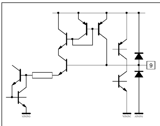
Figure 4 : Pin 9 (YIN)
