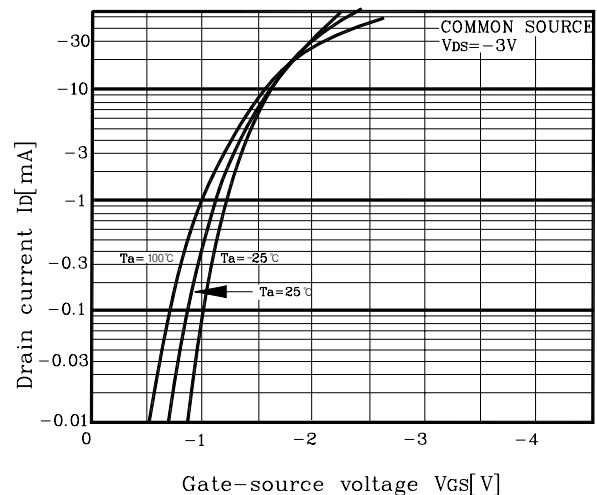
Fig4 I_D - V_{GS}
