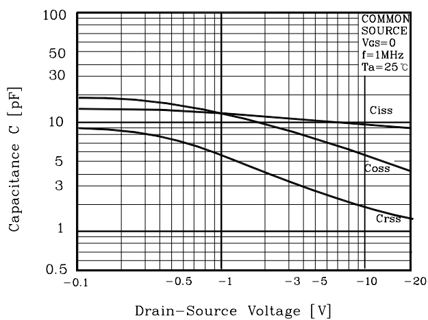
Fig6 C - V_{DS}
