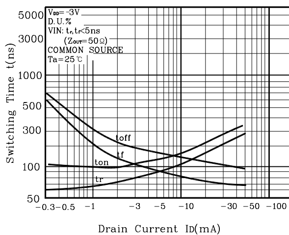
Fig8 t - I_D
