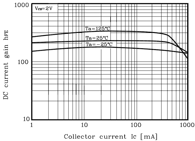
Fig. 7 h_{FE} - I_C
