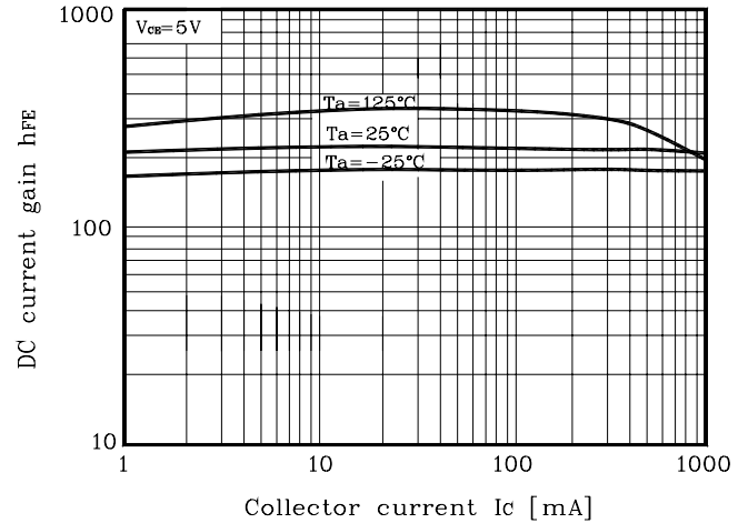
Fig. 8 h_{FE} - I_C
