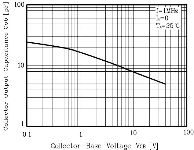
Fig. 9 C_{ob} - V_{CB}
