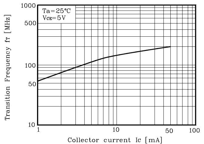
Fig. 10 f_T - I_C
