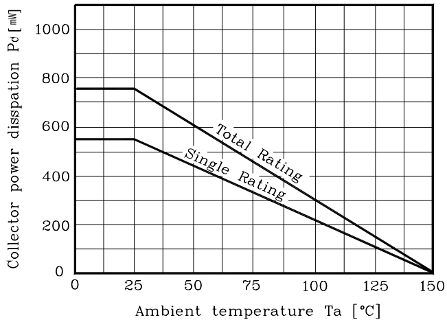
Fig. 1 P_C - T_a
