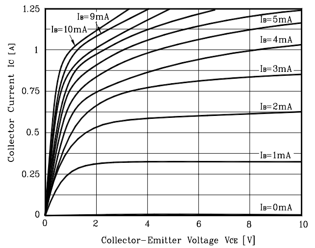
Fig. 8 I_C - V_{CE}
