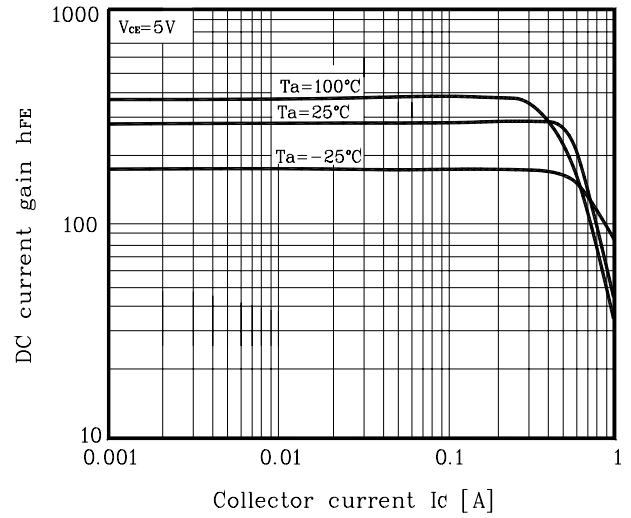
Fig. 8 h_{FE}-I_C
