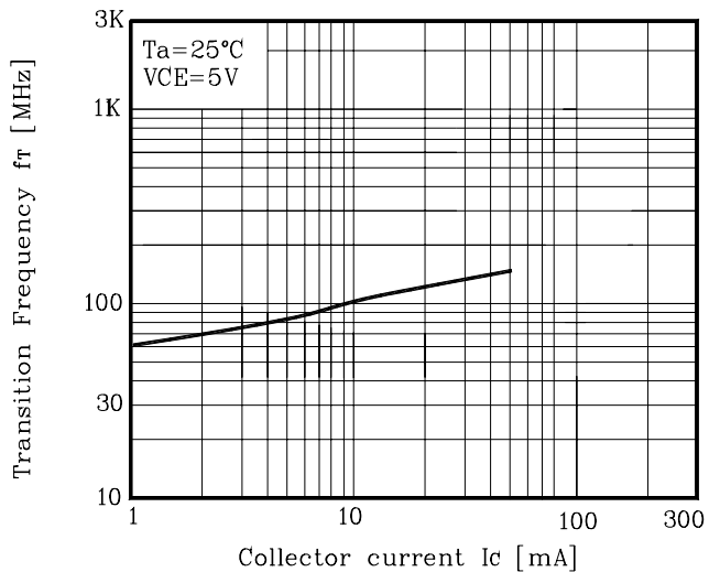
Fig. 11 f_T - I_C
