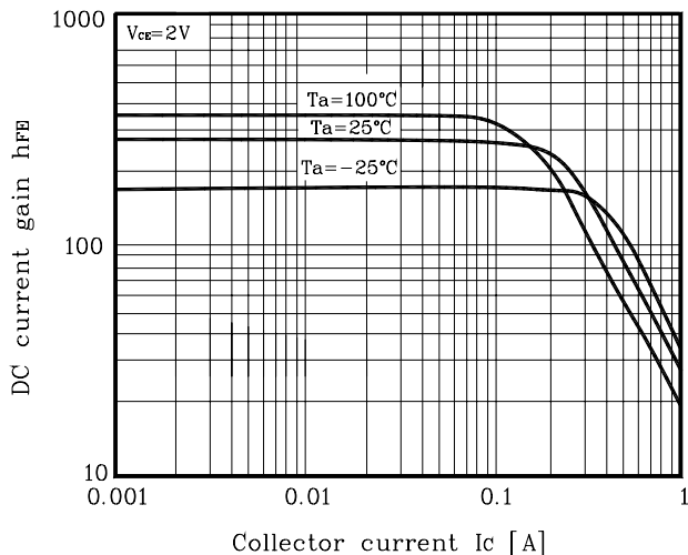
Fig. 9 h_{FE}-I_C
