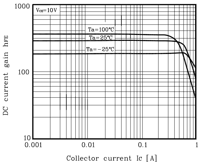
Fig. 9 h_{FE}-I_C
