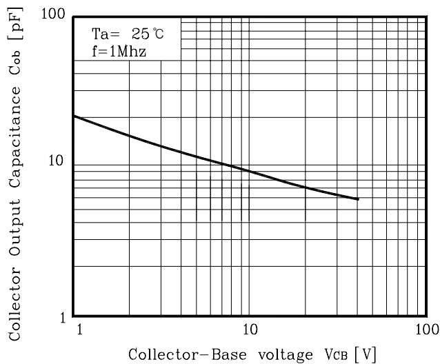
Fig. 10 C_{ob} - V_{CB}
