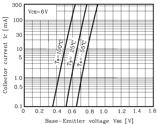
Fig. 1 I_C - V_{BE}
