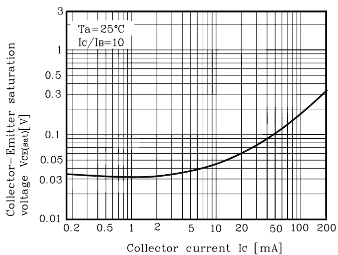
Fig. 4 V_{CE(sat)}-I_C
