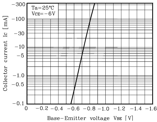
Fig. 1 I_C - V_{BE}
