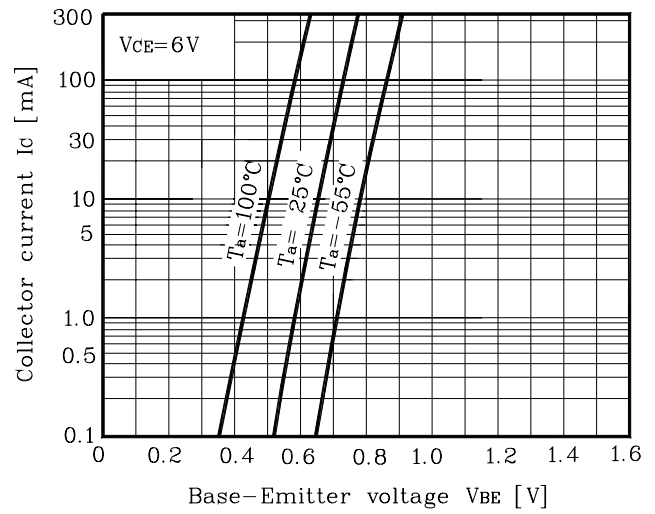
Fig. 2 I_C - V_{BE}
