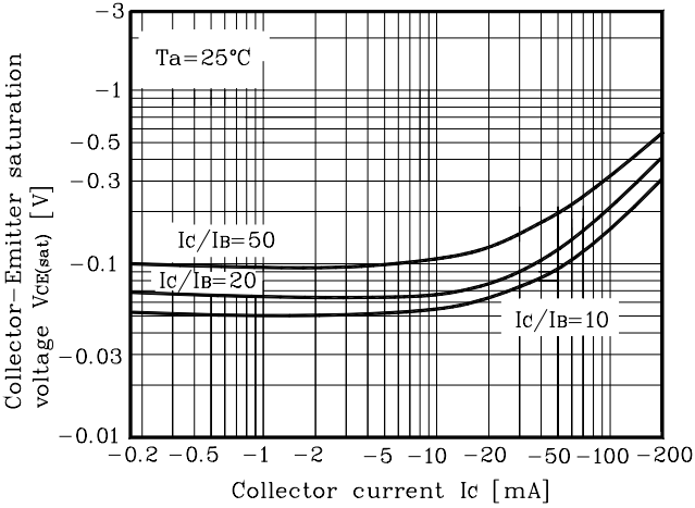
Fig. 4 V_{CE(sat)} - I_C
