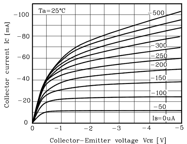
Fig. 2 I_C - V_{CE}
