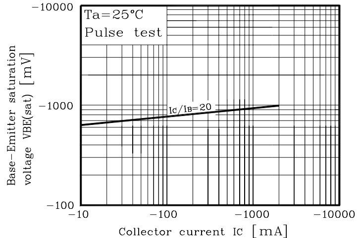
Fig. 6 V_{BE(sat)} - I_C
