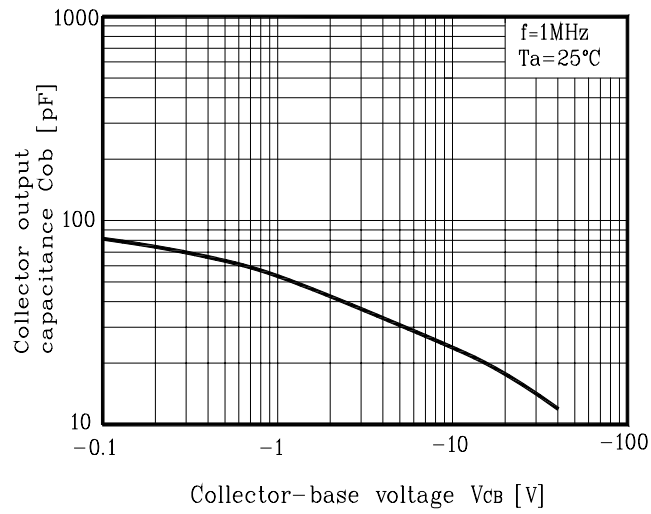
Fig. 7 C_{Ob} - V_{CB}
