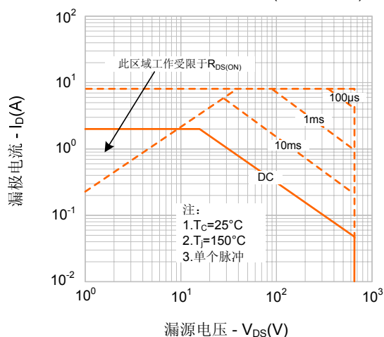
图9-2. 最大安全工作区域(SVF2N65N)
