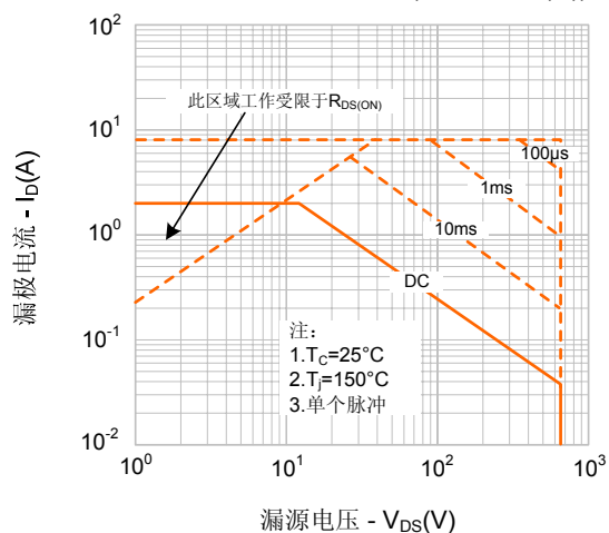
图9-1. 最大安全工作区域(SVF2N65F(G))
