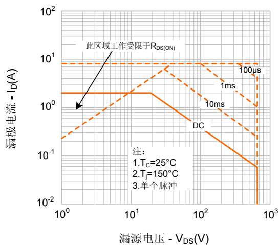
图9-3. 最大安全工作区域(SVF2N65MJ)
