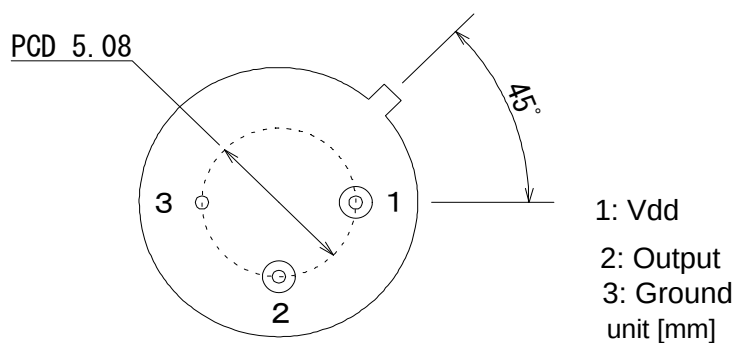
Fig. 1 : Dimensions (Flat package type)
