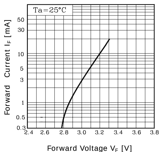
Fig. 1 I_F - V_F
