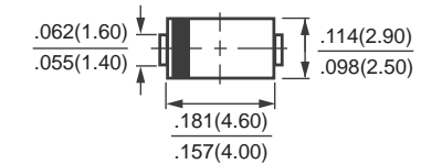
SMA (DO-214AC)
