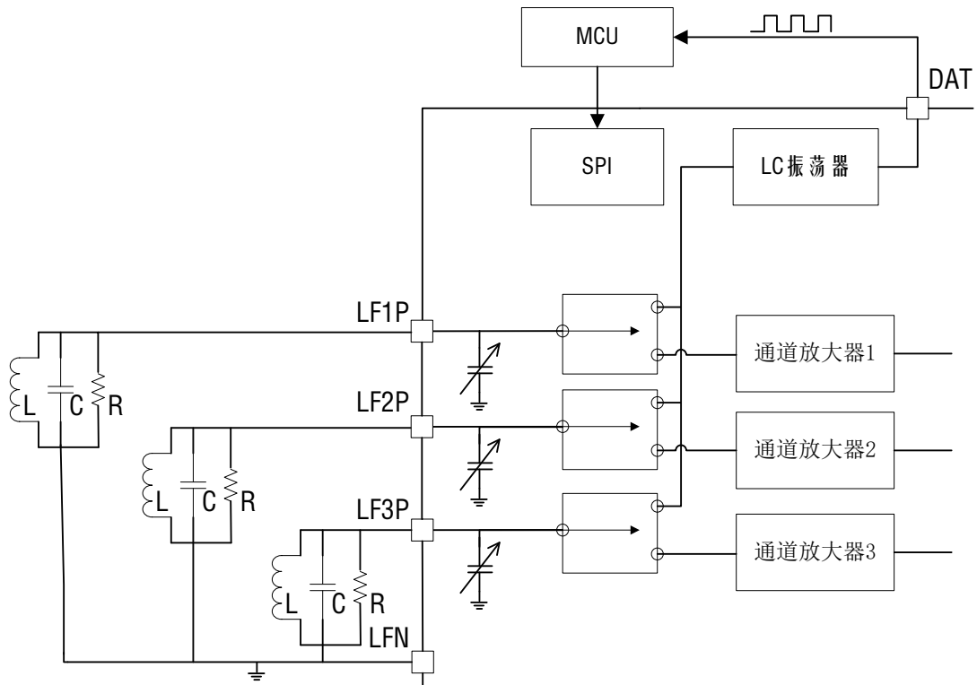
图 7.5-1 天线调谐
