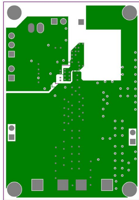
Fig. 44 - Inner Layer 2
