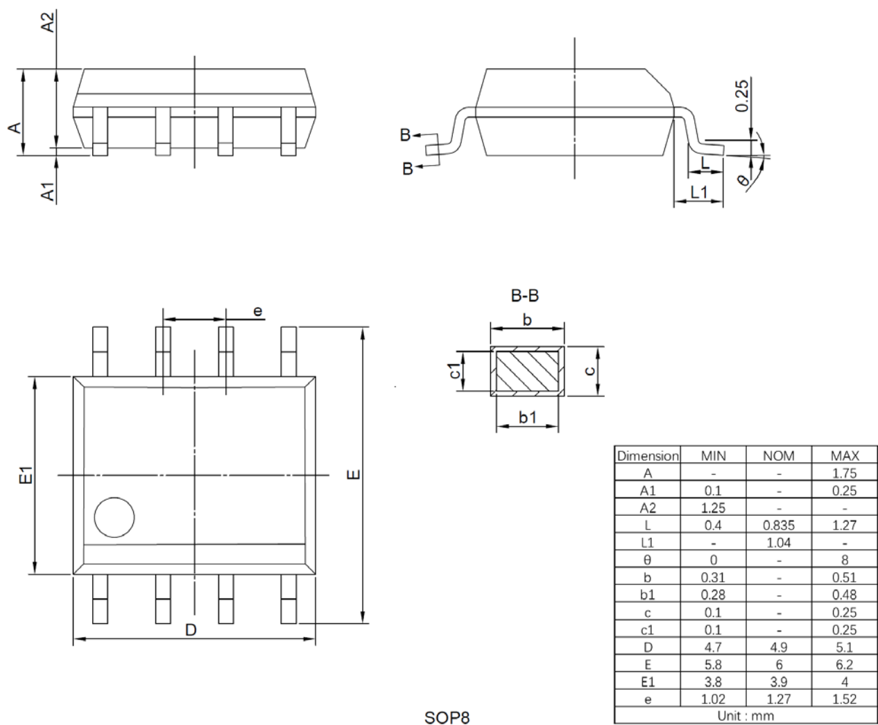
SOP8
